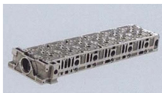
Рис.2. Головка блока цилиндров R6 (масса 136 кг)
